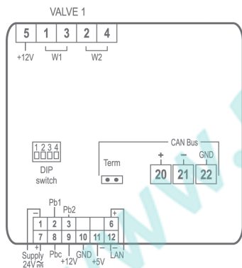
XEV20D - 1 контур
